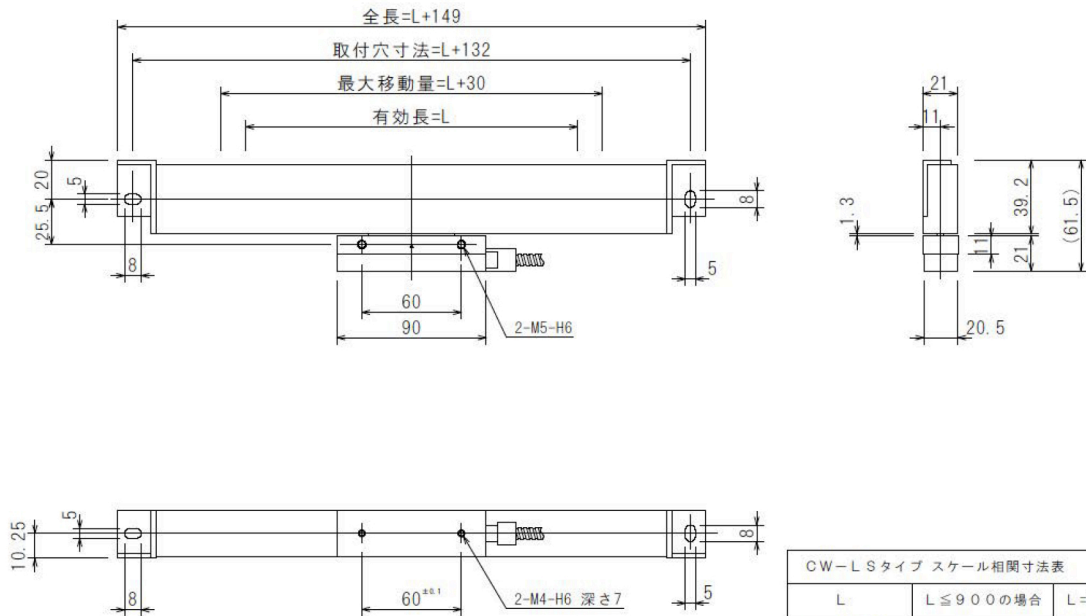
スケール寸法図 <有効長1000mm以下の場合>
