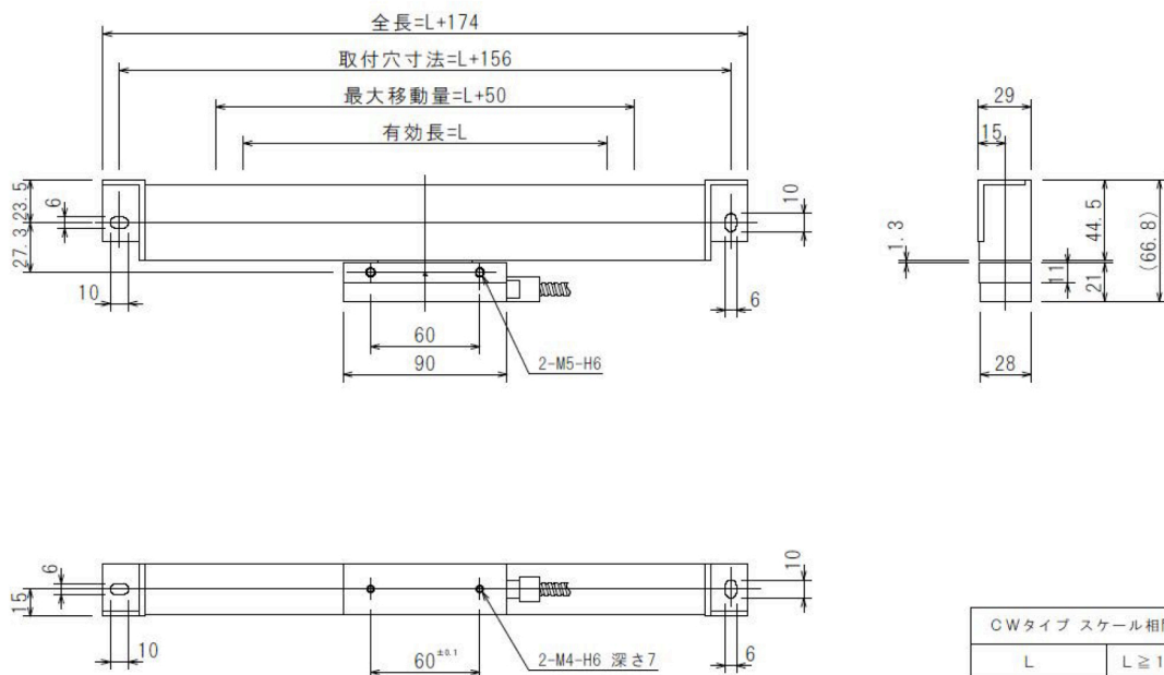
スケール寸法図 <有効長1100mm以上の場合>
